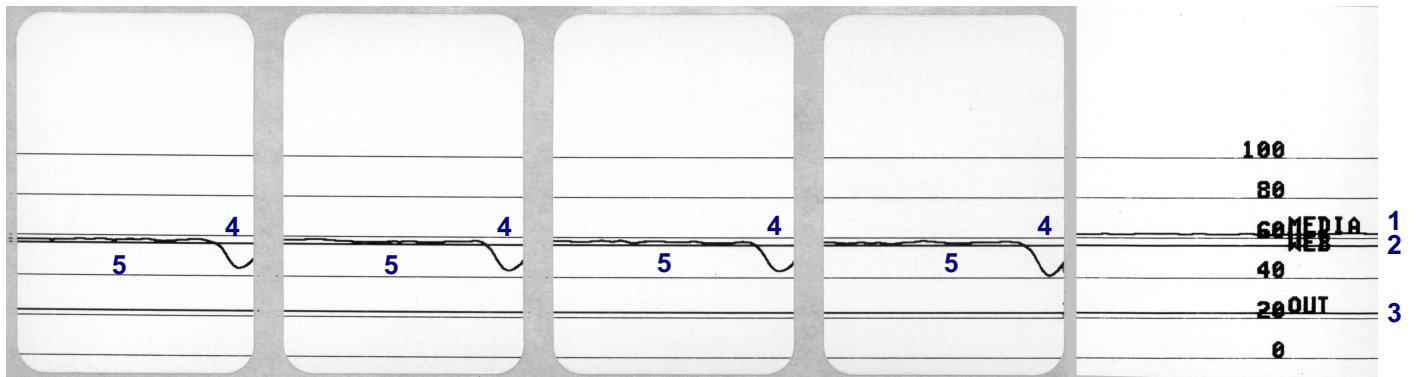
图 22 • 介质传感器校正图 ( 黑色标记介质 )
