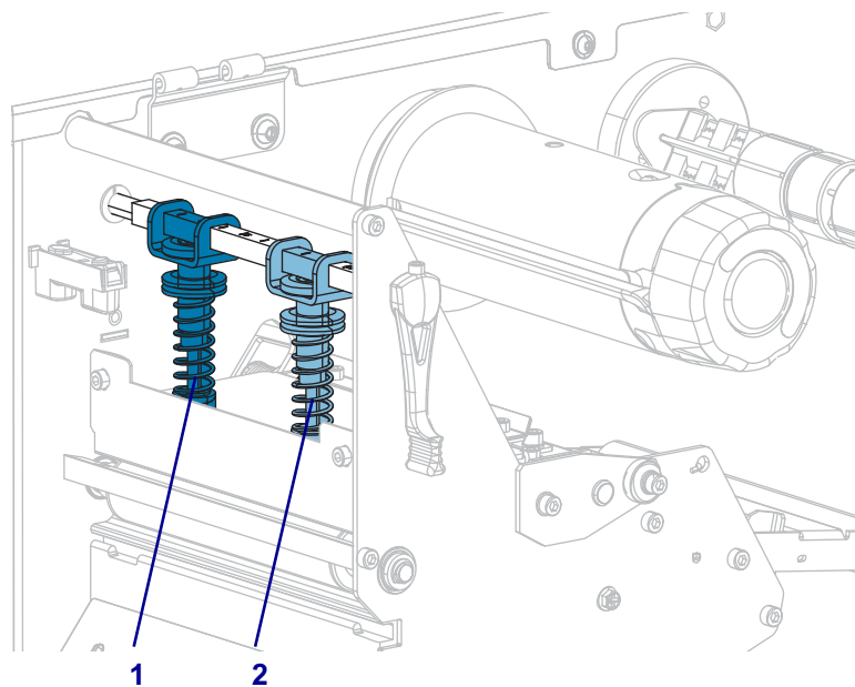
图 17 • 打印头压紧件
