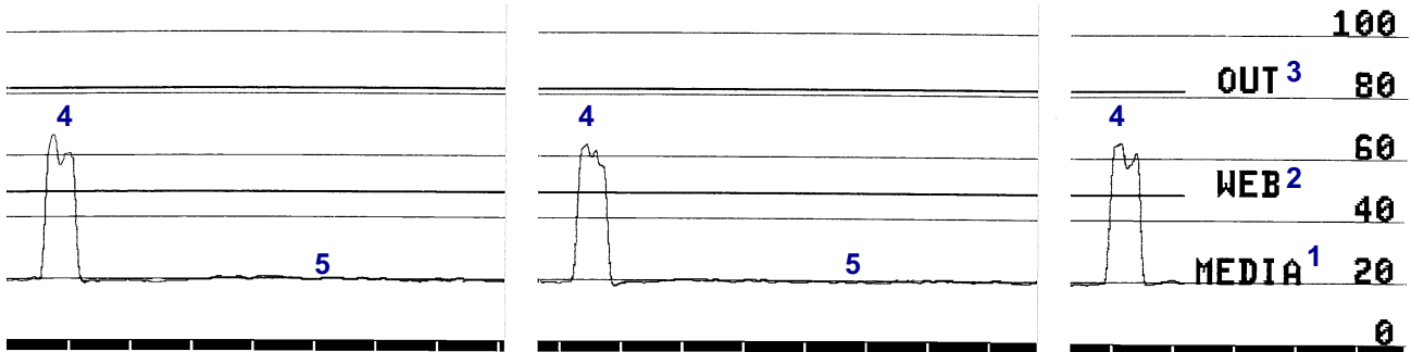
图 21 • 介质传感器校正图 ( 间隙/缺口介质 )
