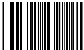
Code 128
